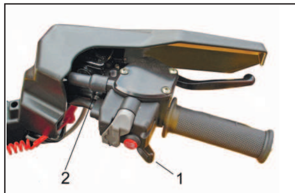
1. Рычаг газа
