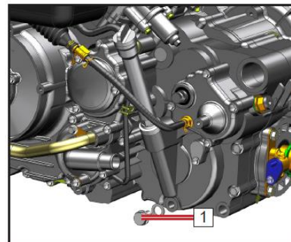
1 Сливная пробка КПП
