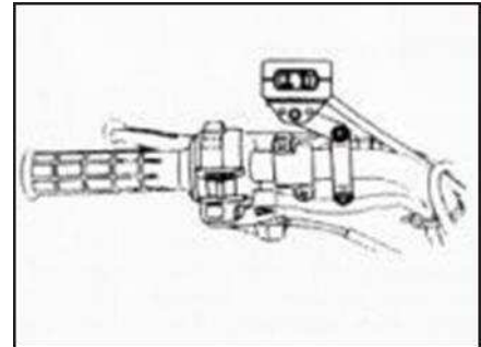
Переключатель, установленный на руле (место и способ установки следует подобрать индивидуально для каждого мотовездехода)
