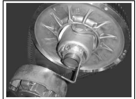
ПРИСПОСОБЛЕНИЕ ДЛЯ РАЗВЕДЕНИЯ ШКИВА В АЛЮМИНИЕВОЙ РЕГУЛИРОВОЧНОЙ МУФТЕ
