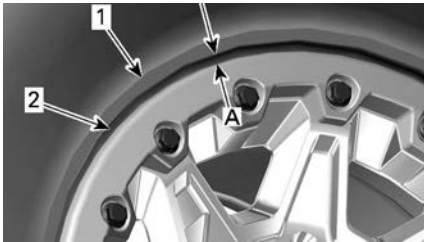
ТИПОВОЙ ВАРИАНТ - ЗАКЛЮЧИТЕЛЬНЫЙ ЭТАП ЗАТЯЖКИ ВИНТОВ
