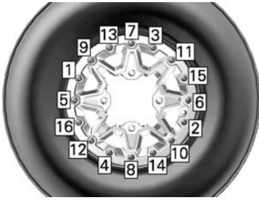
ТИПОВОЙ ВАРИАНТ - ПОРЯДОК ЗАТЯЖКИ ВИНТОВ
