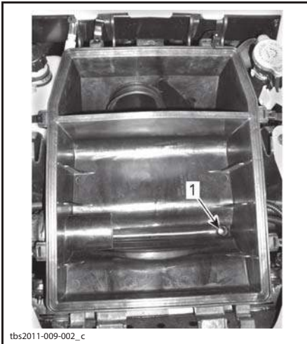
1. Сливное отверстие
