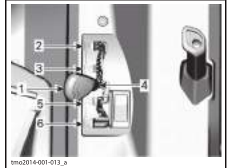
1. Рычаг переключения передач 2. Парковочная блокировка 3. Передача заднего хода 4. Нейтраль 5. Повышенная передача (при движении вперед) 6. Пониженная передача (при движении вперед)
