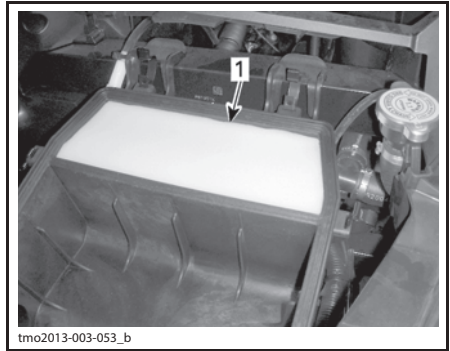
1. Дополнительный фильтрующий элемент воздушного фильтра двигателя
