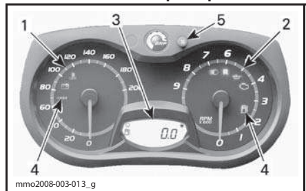
АНАЛОГОВАЯ/ЦИФРОВАЯ ПАНЕЛЬ ПРИБОРОВ (СТАНДАРТНЫЙ ВАРИАНТ)
