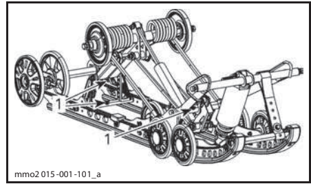
1. Пресс-масленки
