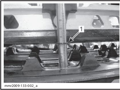
1. Нижнее кольцо вровень с нижней кромкой накладки полаза
