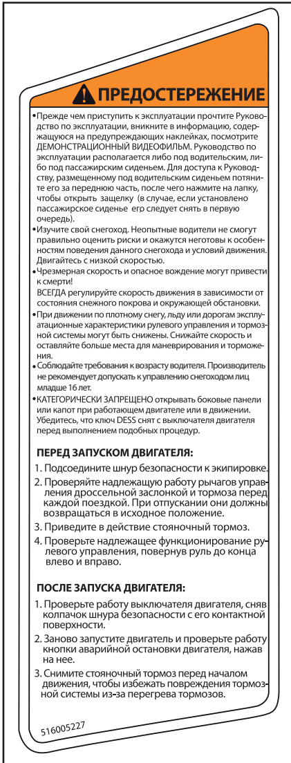
НАКЛЕЙКА 8
