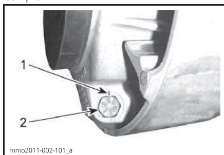
РЕГУЛИРОВКА ШКИВА
