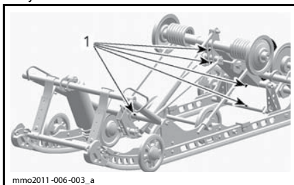
1. Пресс-масленка
