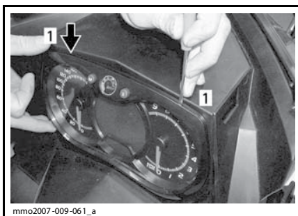
1. Защелка
