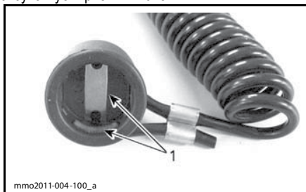
КОЛПАЧОК ШНУРА БЕЗОПАСНОСТИ 1. Отсутствует снег или грязь
