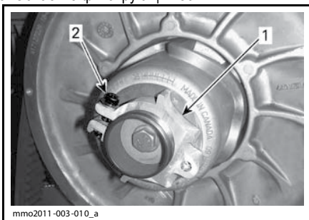
1. Регулировочная муфта
