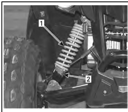
DS 70 и DS 90 — ПЕРЕДНЯЯ ПОДВЕСКА
