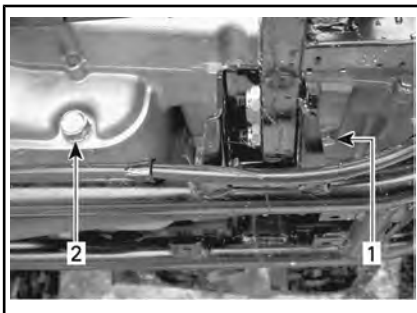
ПРОБКА СЛИВНОГО ОТВЕРСТИЯ — ЛЕВАЯ СТОРОНА ДВИГАТЕЛЯ
