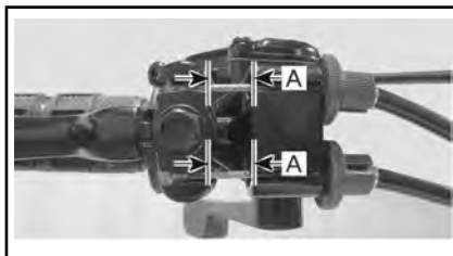
1. Регулировочные винты на рычаге тормоза
