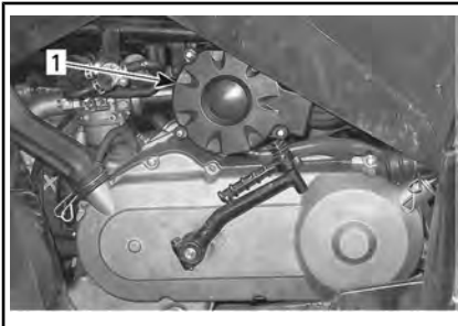
ЛЕВАЯ СТОРОНА СТОРОНА ТРАНС- ПОРТНОГО СРЕДСТВА
