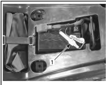
1. Держатель предохранителей.
