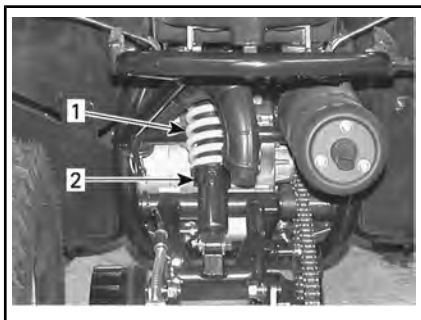
DS 70 and DS 90 — ЗАДНЯЯ ПОДВЕСКА
