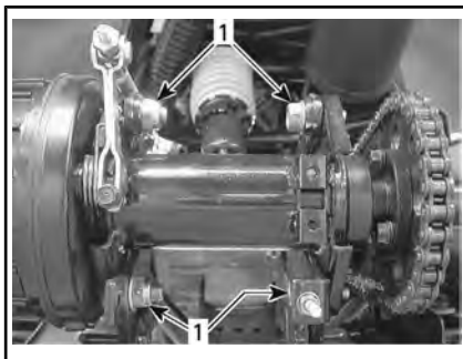
ТИПОВОЙ ВАРИАНТ — ЗАДНИЙ МОСТ
