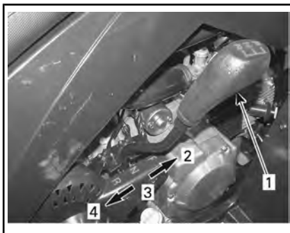
СХЕМА ПЕРЕКЛЮЧЕНИЯ ПЕРЕДАЧ
