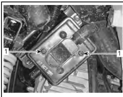
1. Выверните винты
