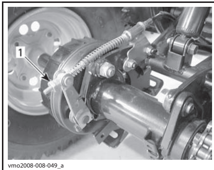
1. Регулировочная муфта
