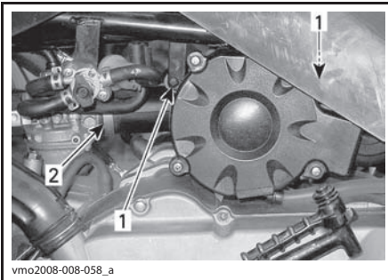
1. Выверните винты 2. Отпустите хомут
