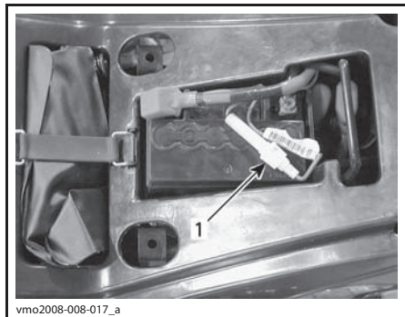
1. Держатель предохранителя
