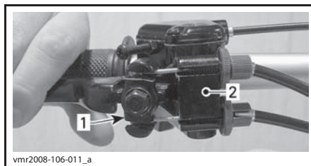
1. Шарнир троса
