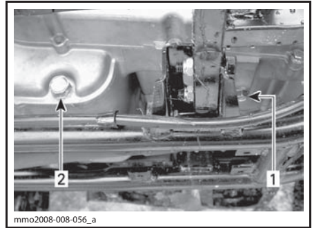
1. Пробка сливного отверстия коробки передач 2. Сливная пробка картера двигателя
