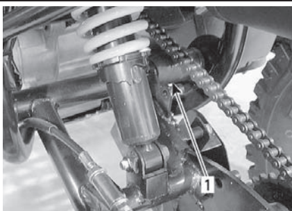
1. Ролик приводной цепи
