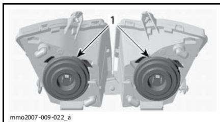
1. Резиновые кожухи
