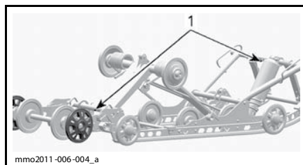
1. Пресс-масленки
