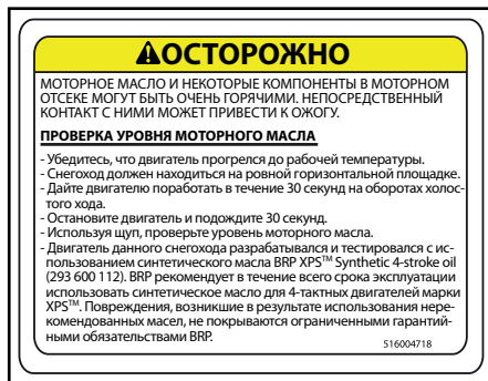
МОДЕЛЬ 1200 4-ТЕС - В МОТОРНОМ ОТСЕКЕ
