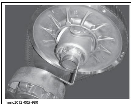
ПРИСПОСОБЛЕНИЕ ДЛЯ РАЗВЕДЕНИЯ ВЕДОМОГО ШКИВА УСТАНОВЛЕНО В АЛЮМИНИЕВУЮ РЕГУЛИРОВОЧНУЮ МУФТУ
