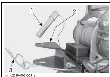
1. Палец 2. Монтажные пластины 3. Шплинт
