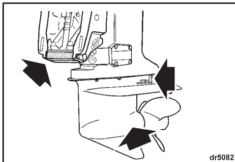
1. Модели с автоматическим подъемом и тримом — точки смазки транспортировочного кронштейна и кронштейна подъема (смазывать ежегодно)
