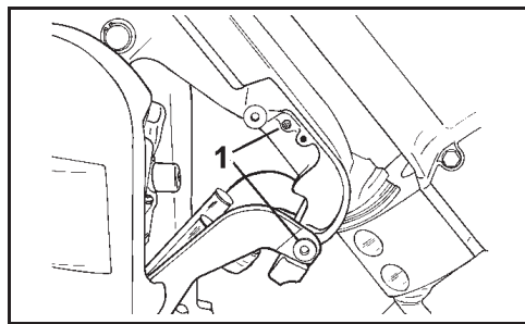
1. Модели с автоматическим подъемом и тримом — точки смазки транспортировочного кронштейна и кронштейна подъема (смазывать ежегодно)
