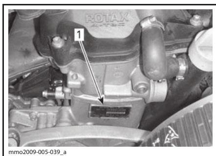
ДВИГАТЕЛЬ 1200 4-TEC
