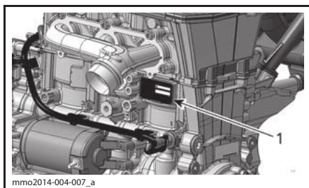
ДВИГАТЕЛЬ 900 ACE
