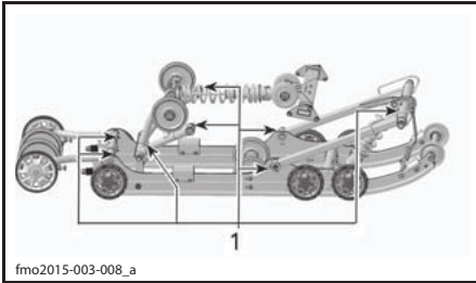
1. Пресс-масленки
