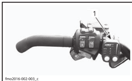
1. Модуль ECS 2
