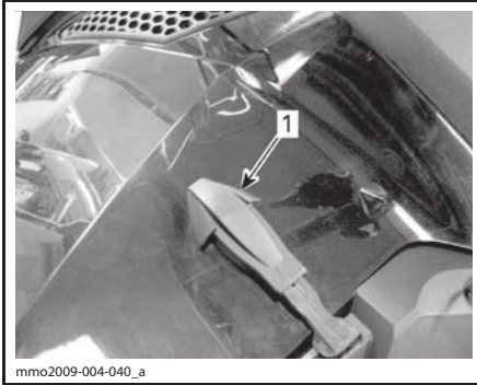
1. Резиновый фиксатор
