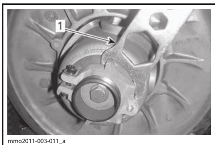
АЛЮМИНИЕВАЯ РЕГУЛИРОВОЧНАЯ МУФТА 1. Приспособление для регулировки
