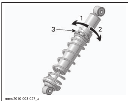
РЕГУЛЯТОР КУЛАЧКОВОГО ТИПА — АМОРТИЗАТОР НРР
