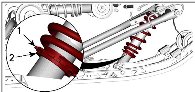
1. Регулировочное кольцо 2. Стопорное кольцо
