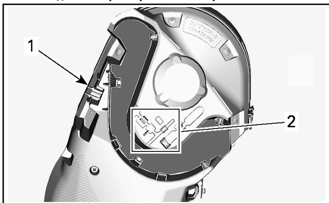
ЗАЩИТНЫЙ КОЖУХ РЕМНЯ ВАРИАТОРА
