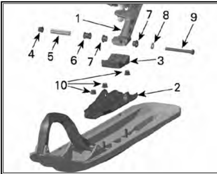
РАСПОЛОЖЕНИЕ КОМПОНЕНТОВ — ПОКАЗАНА ПРАВАЯ СТОРОНА
