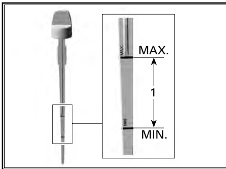
1. Уровень масла между метками «MIN» и «MAX»
