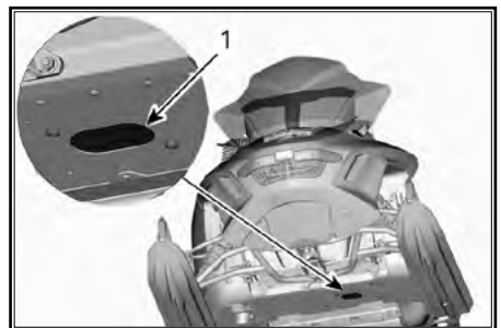
1. Крышка отверстия, обеспечивающего доступ к пробкам сливных отверстий
