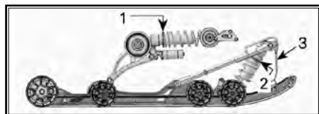
ТИПОВОЙ ВАРИАНТ — PPS2 — РЕГУЛИРУЕМЫЕ КОМПОНЕНТЫ
