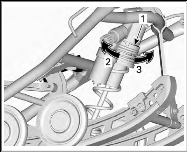
ТИПОВОЙ ВАРИАНТ — РЕГУЛЯТОР КОЛЬЦЕВОГО ТИПА 1. Регулировочное кольцо предварительного натяжения пружины 2. Увеличить предварительный натяг 3. Уменьшить предварительный натяг
