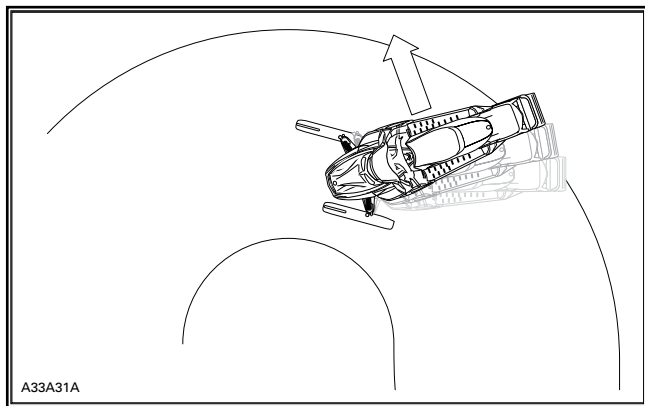
ИЗБЫТОЧНАЯ ПОВОРАЧИВАЕМОСТЬ
