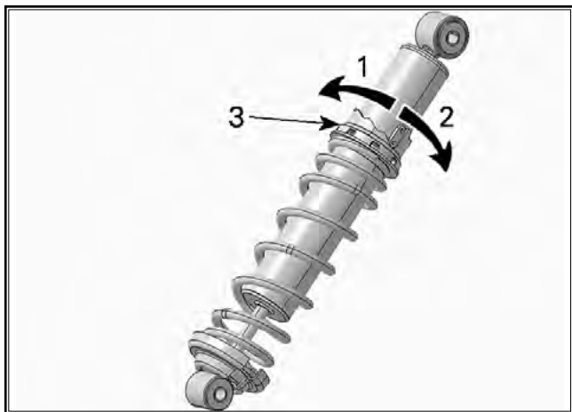
РЕГУЛЯТОР КУЛАЧКОВОГО ТИПА — АМОРТИЗАТОР NPG
