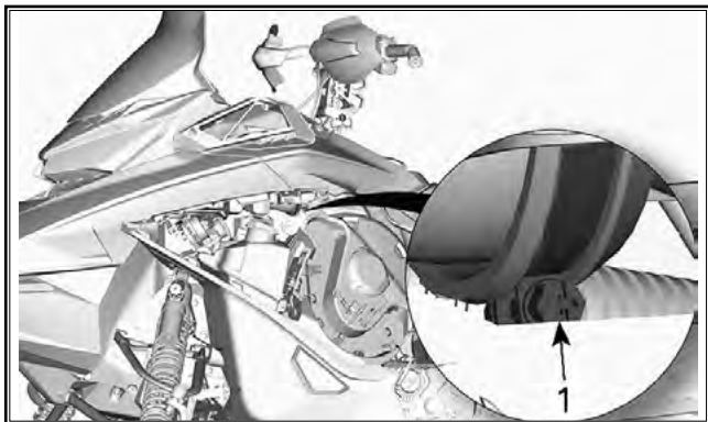
1. Хомут
