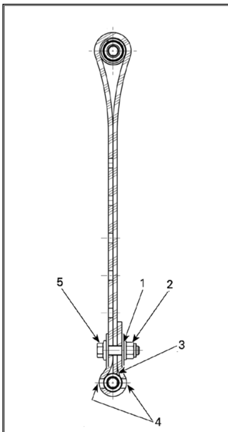
ЛЕНТОЧНЫЙ ОГРАНИЧИТЕЛЬ В ПОЛОЖЕНИИ 1 (ПЕРВОЕ ОТВЕРСТИЕ, САМАЯ БОЛЬШАЯ ДЛИНА)
