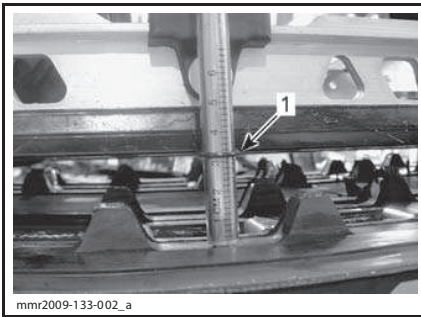
1. Нижнее кольцо вровень с нижней кромкой накладок полоза
