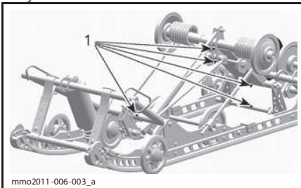
1. Пресс-масленки
