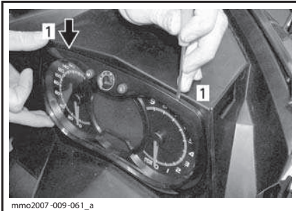
1. Защелка
