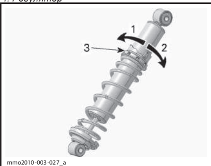
ТИП РЕГУЛЯТОРА - АМОРТИЗАТОР С ГАЗОВЫМ ПОДДОРОМ ВЫСОКОГО ДАВЛЕНИЯ (НРГ) 1. Уменьшение преднатяга 2. Увеличение преднатяга 3. Регулятор преднатяга пружины
