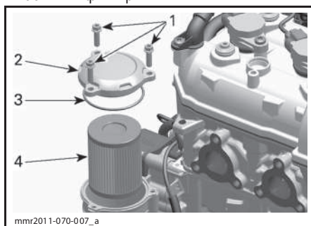
mmr2011-070-007_a 1. Винты крышки масляного фильтра 2. Крышка масляного фильтра 3. Кольцевое уплотнение 4. Масляный фильтр
