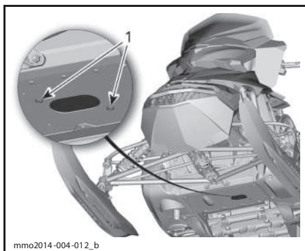
ПОВЕРНИТЕ СЕРВИСНУЮ КРЫШКУ 1. Фиксирующие винты
