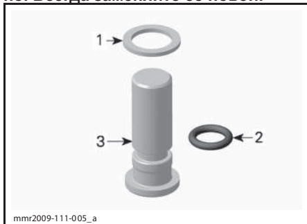
mmr2009-111-005_a 1. Уплотнительная шайба 2. Кольцевое уплотнение 3. Сливная пробка
