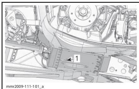
mmr2009-111-101_a 1. Отверстие в раме для доступа к сливной пробке
