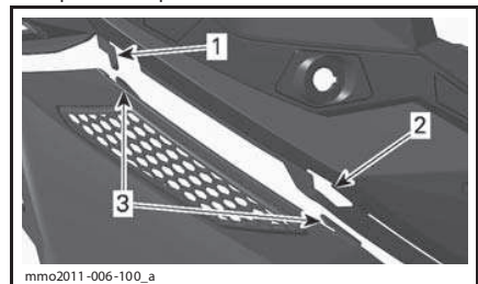
1. Крюк консоли 2. Отверстие консоли 3. Верхние лапки панели
