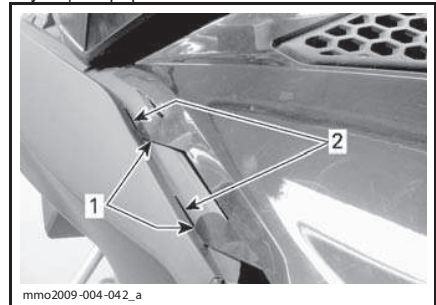
1. Нижние лапки панели 2. Прорези нижнего поддона
