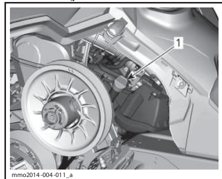
ЛЕВАЯ СТОРОНА СНЕГОХОДА 1. Щуп в масляном баке
